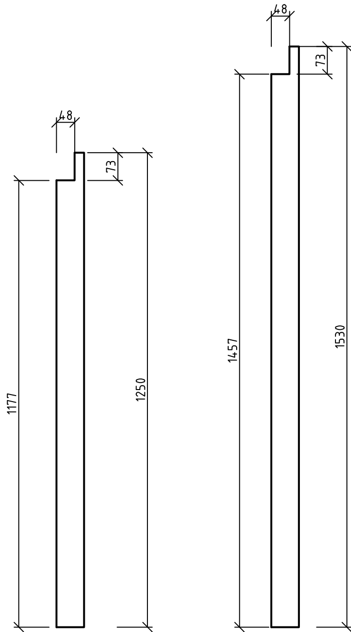
Pystytolpat 48x73 HS
